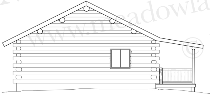
RIGHT ELEVATION
