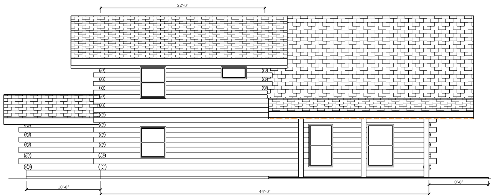
RIGHT ELEVATION
