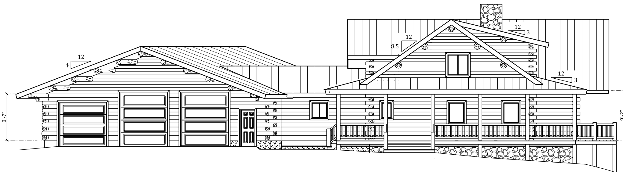
RIGHT ELEVATION
