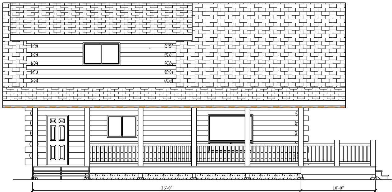
RIGHT ELEVATION
