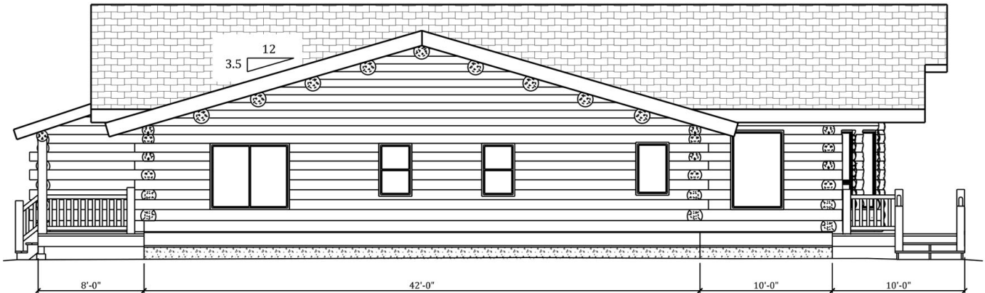
RIGHT ELEVATION
