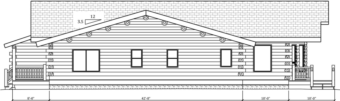
RIGHT ELEVATION
