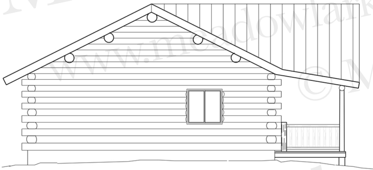
RIGHT ELEVATION
