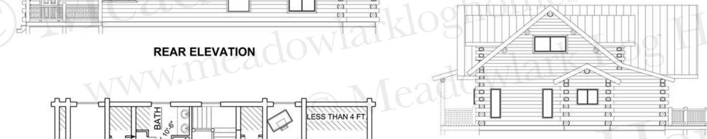
RIGHT ELEVATION
